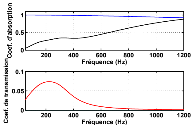
FIGURE 8 – Coefficient d'absorption (sans contrôle : noir, avec contrôle bleu) et module du coefficient de transmission (sans contrôle : rouge, avec contrôle cyan) de la cellule hybride double.
