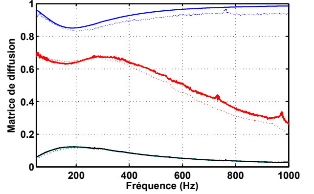
FIGURE 5 – Matrice de diffusion de la cellule hybride en circuit ouvert. D_{11} : rouge, D_{22} : bleu, D_{12} : cyan et D_{21} : noir. Mesure : pointillés, "modélisation" : trait plein.
